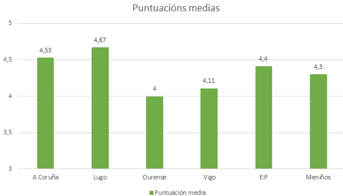
Figura 1. Puntuacións medias.
